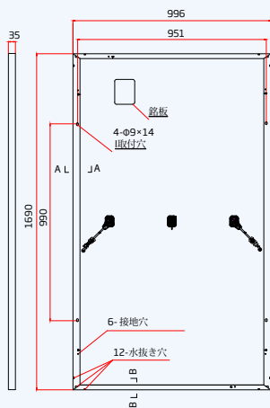
背面図
